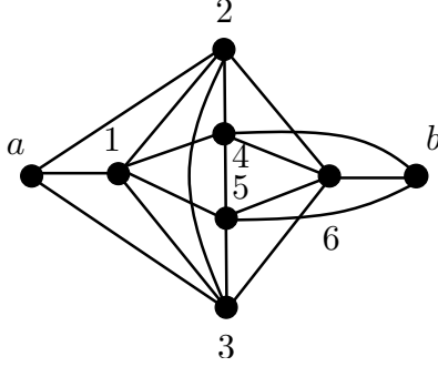
Fig. 3. The triple edge gadget.
