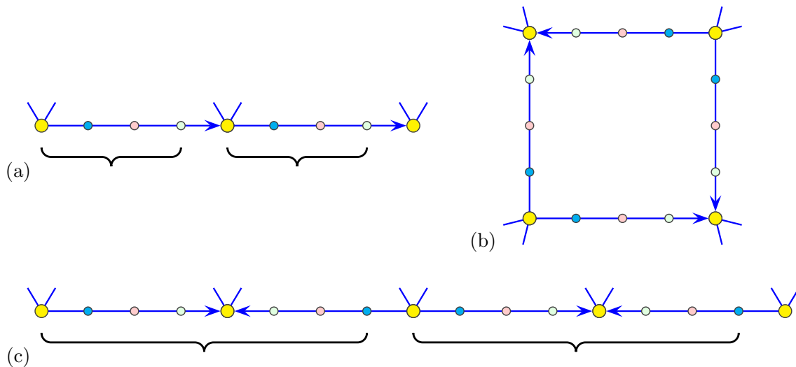
FIGURE 7. Illustration for Lemma 9.12.
